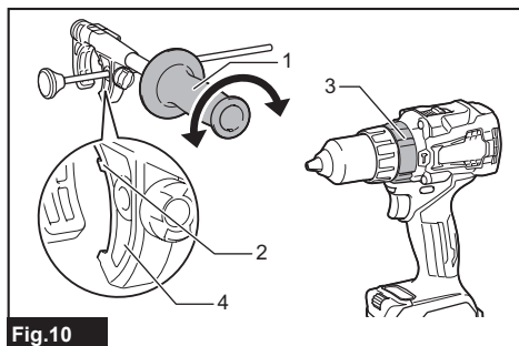
Fig.10 ► 1. Side grip 2. Protrusion 3. Groove 4. Arm
